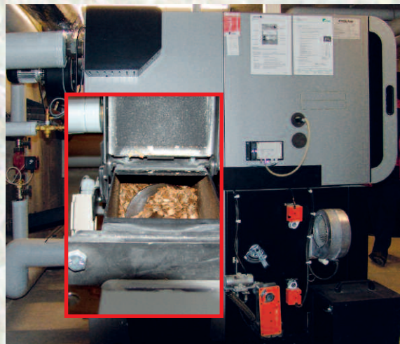
Holzhackschnittel-Heisanlage im Naturfreundehaus Sommerecke
